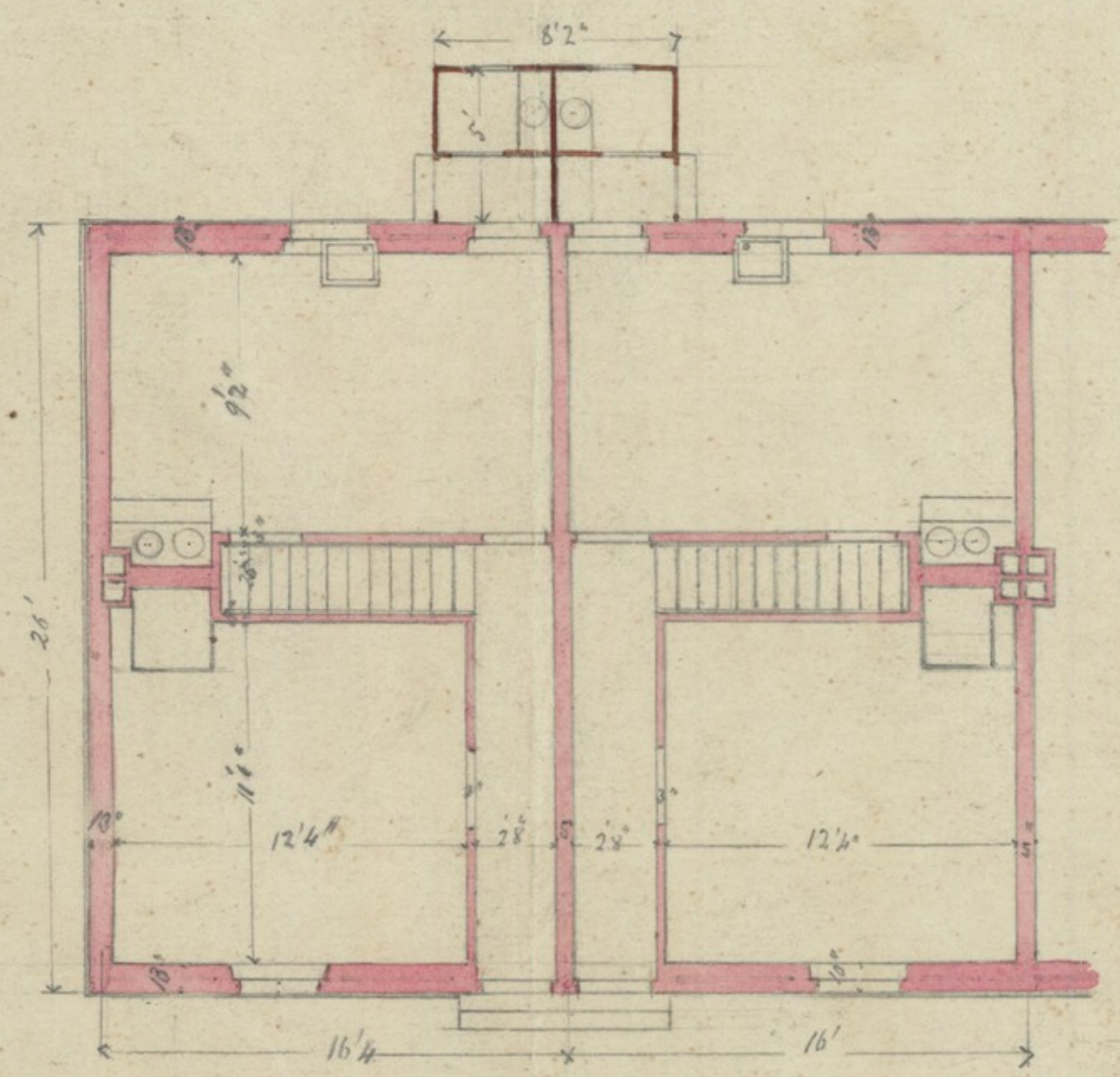
Erdgeschoss
