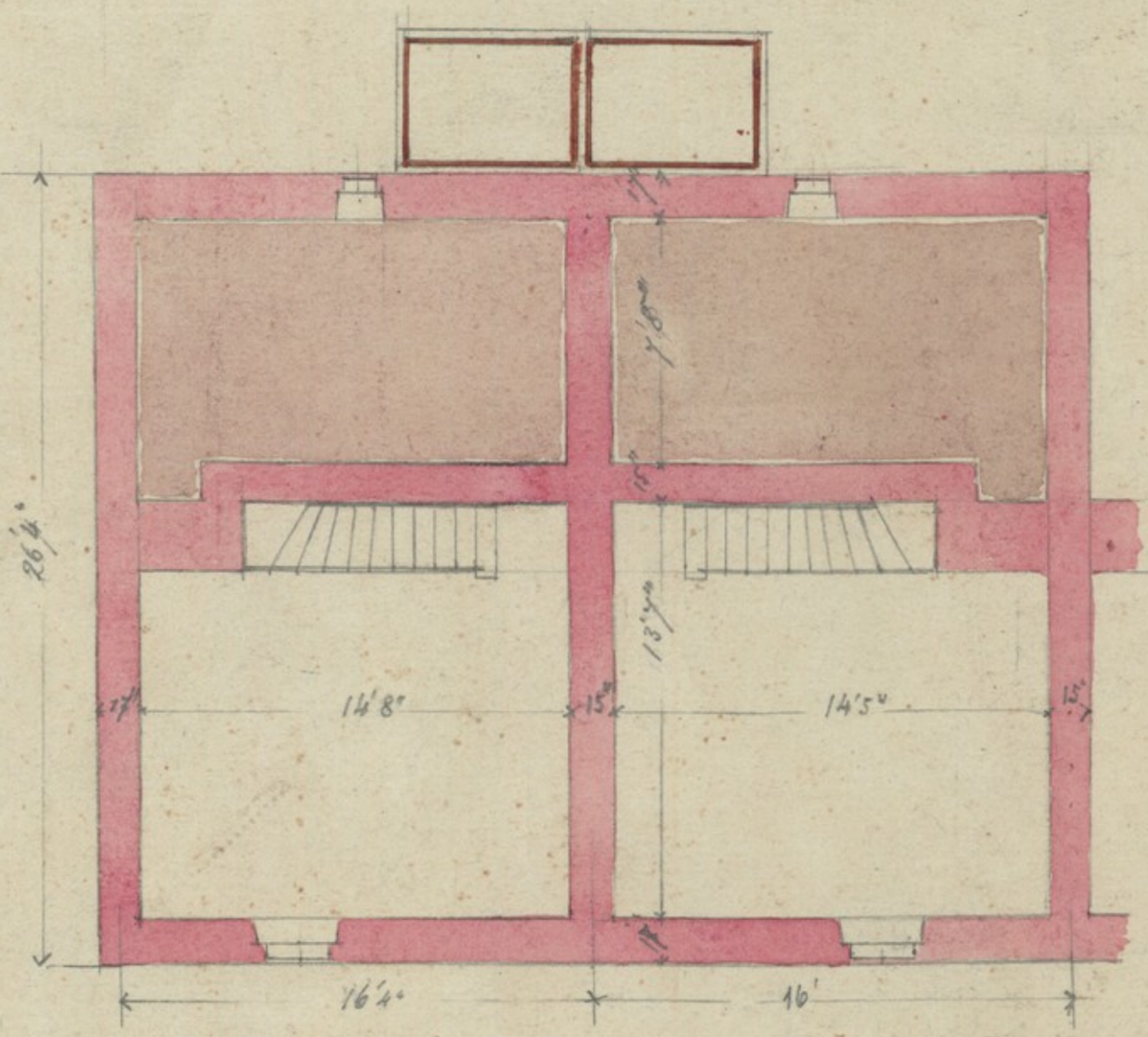
Kellergrundriss
